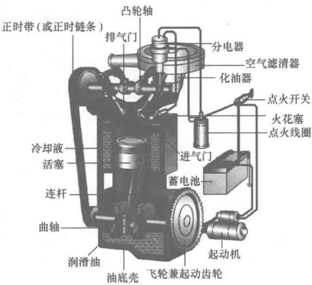
图 1-2 发动机的总体构造
