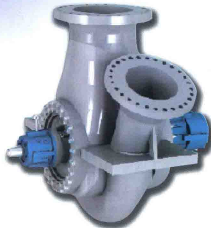
前置泵
