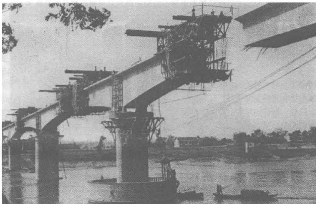
图 1-3 悬臂灌注法施工
