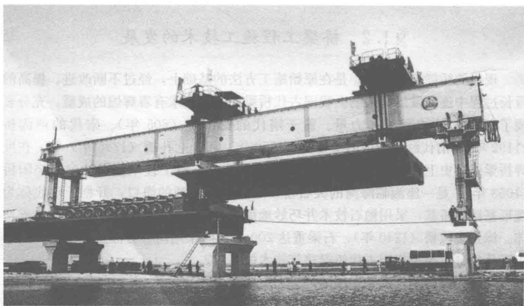
图 1-1 JQ600 架桥机架梁
