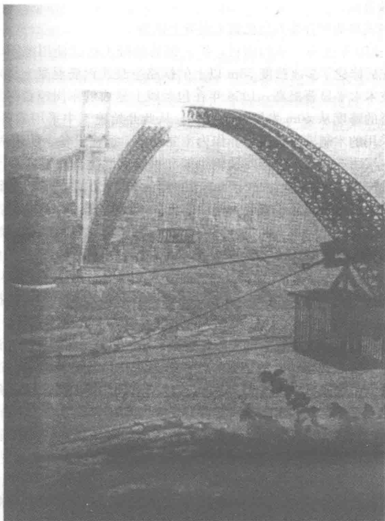
图 1-2 混凝土拱桥劲性骨架吊装
