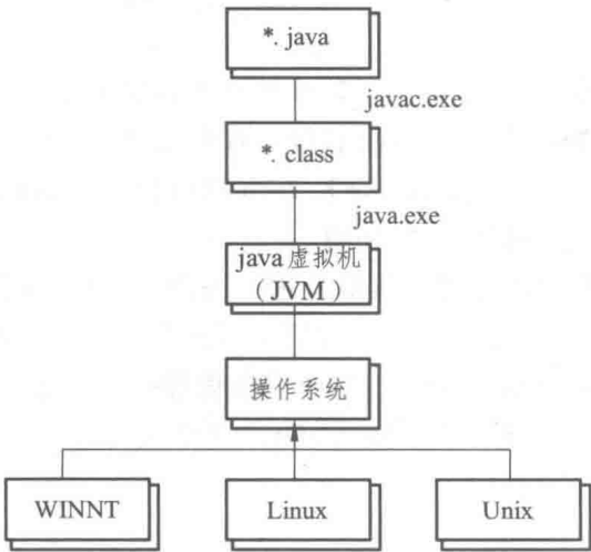
图 1-1 Java 虚拟机
