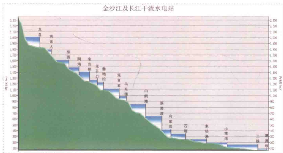
▲ 图 29 从龙盘峡到葛洲坝阶梯电站剖面图
