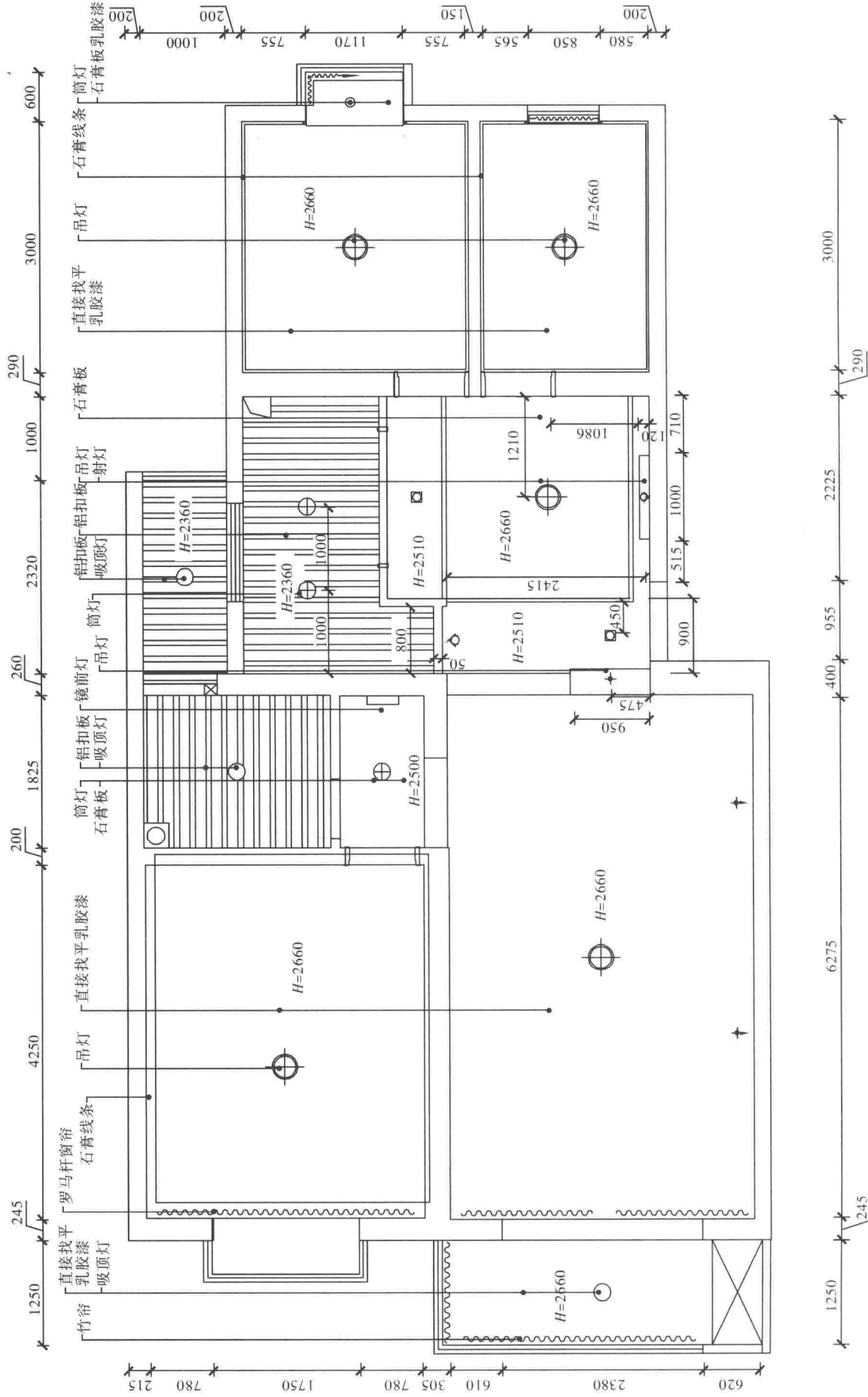
天花布置图 1:40
