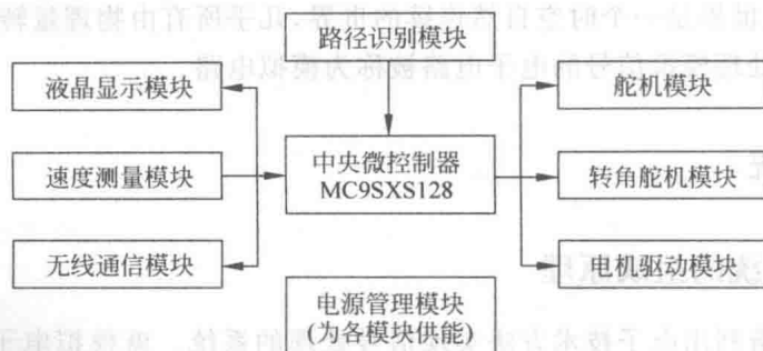
图 1.1 控制系统框图
