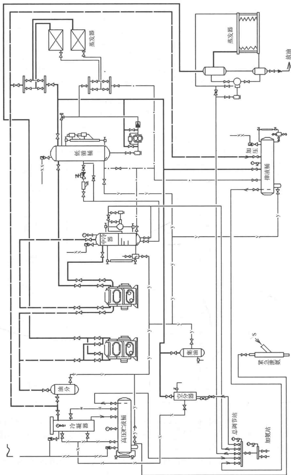
图 1-1-5 常见的冷库制冷系统原理
