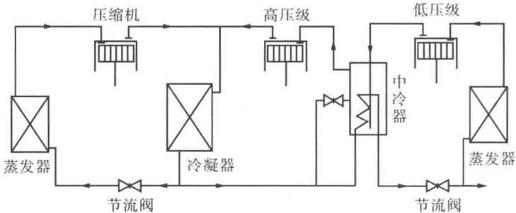
图 1-1-3 单、双级压缩综合系统基本构成
