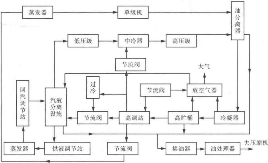
图 1-1-4 单、双级综合系统制冷流程
