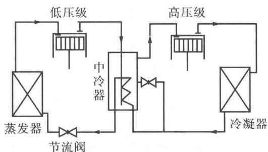
图 1-1-2 双级压缩系统基本构成
