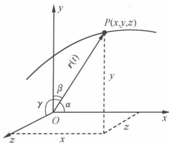
图 1-1 质点位置的坐标和位矢
