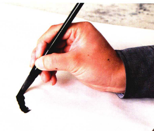
侧锋运笔
