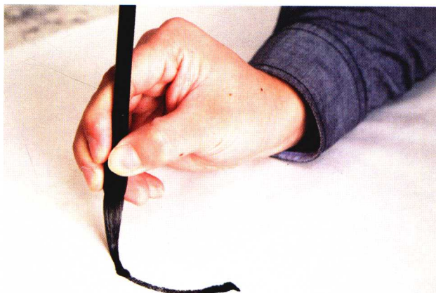
中锋运笔 2
