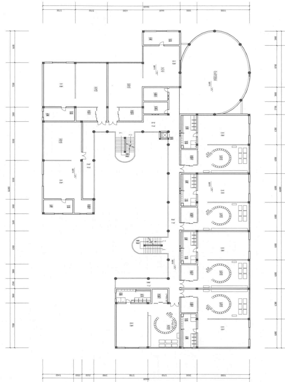
四层平面图
