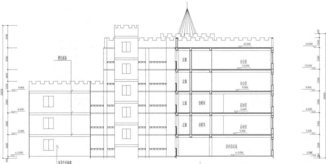
剖面图
