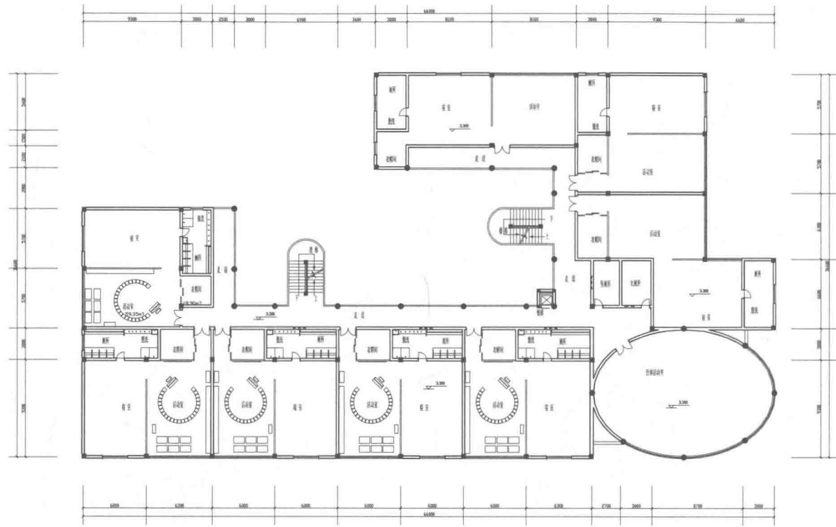
二层平面图
