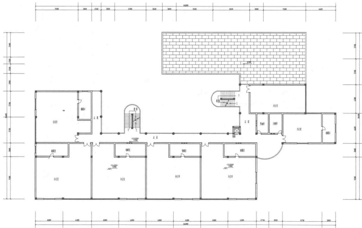
三层平面图
