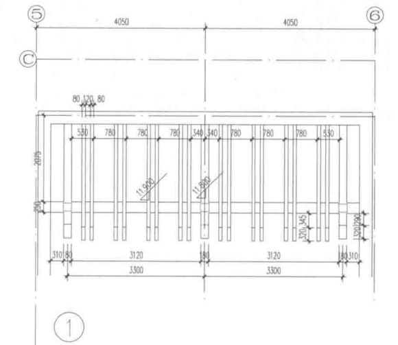
屋顶平面图
