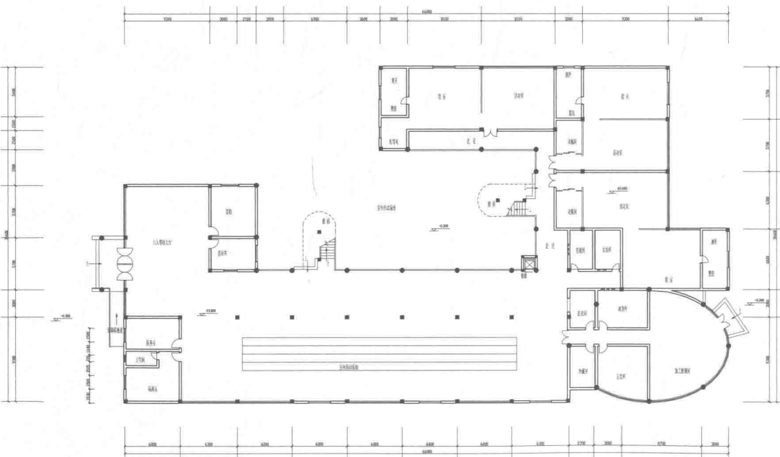
一层平面图
