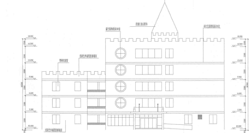
剖面图
