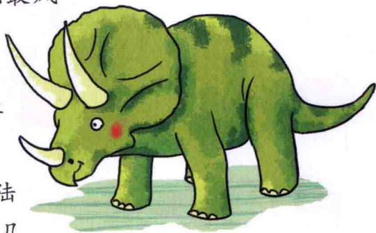
三角龙
