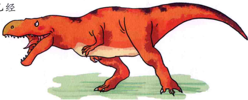
霸王龙
