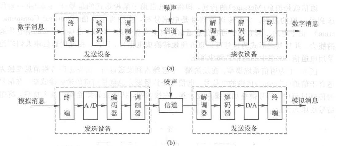
图 0-3 数字通信系统模型
