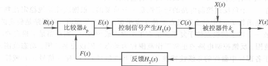
图 1-2 反馈控制电路的 s 域数学模型
