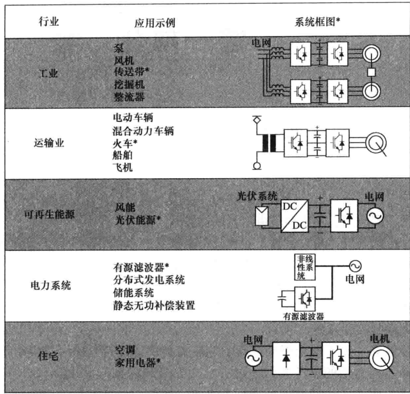
图 1.1 功率变换器的应用
