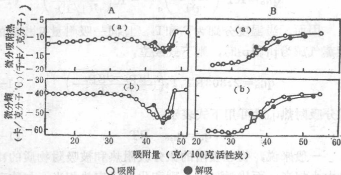
图 1-1 吸附苯时的微分吸附热及微分熵
