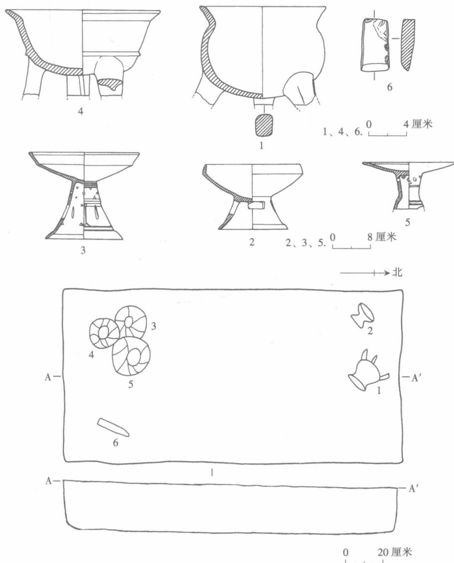
图七 96M5 平剖面图及随葬器物
