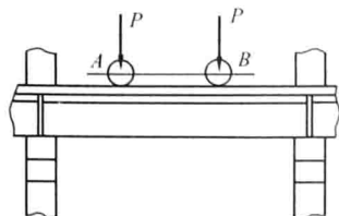
图 1-7 吊车梁
