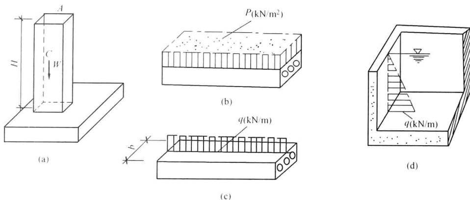
图 1-5 荷载的分布形式
