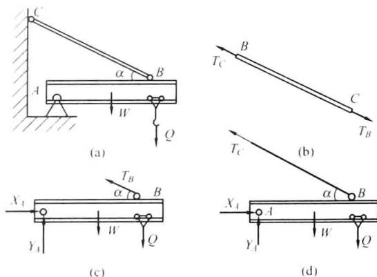
图 1-16 [例 1-2] 图
