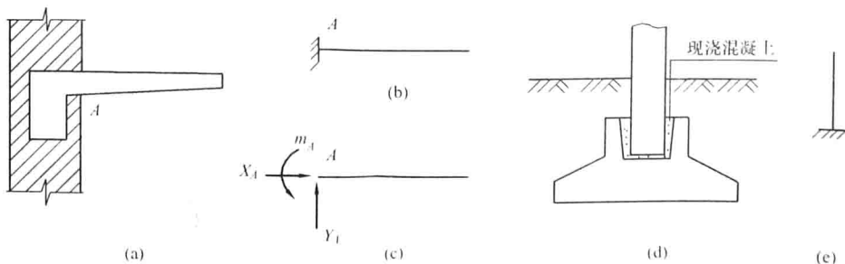
图 1-14 固定端支座及其反力
