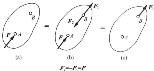
图 1-3 力的可传性
