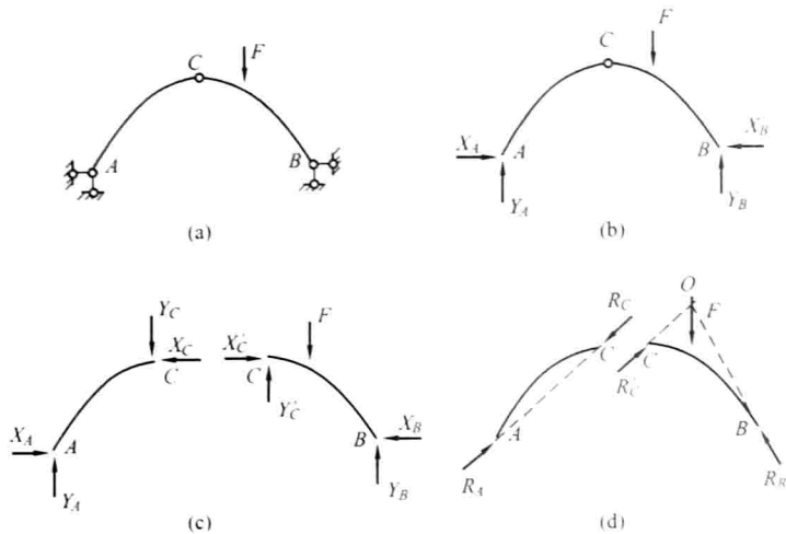
图 1-17 [例 1-3] 图
