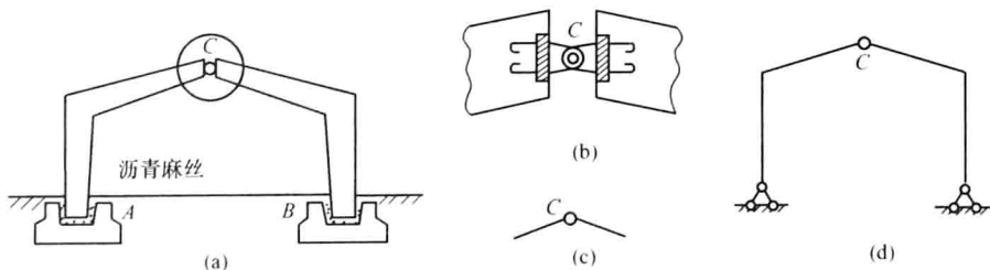
图 1-10 结构的铰链联结
