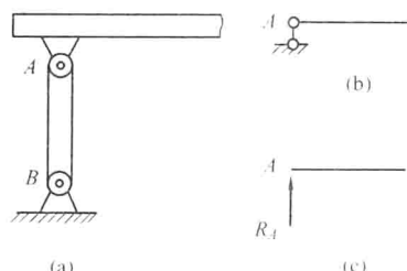
图 1-13 单链杆支座及其反力
