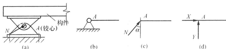
图 1-11 固定铰链约束及其反力
