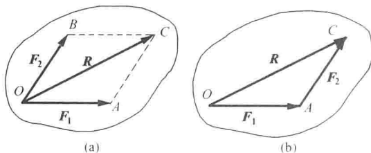
图 1-4 力的平行四边形、三角形法则
