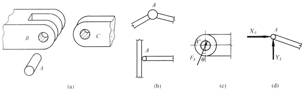
图 1-9 光滑铰链约束及其反力
