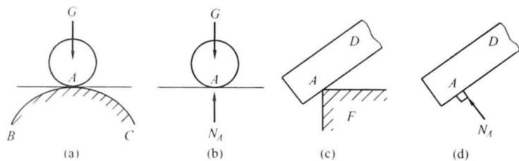
图 1-8 光滑接触面约束及其反力
