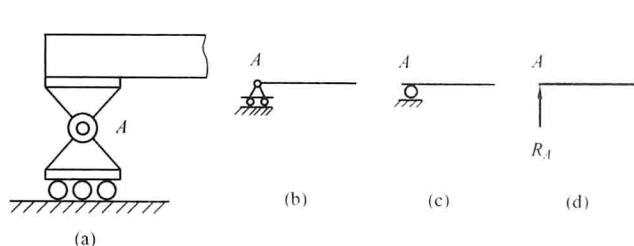
图 1-12 可动铰链支座及其反力
