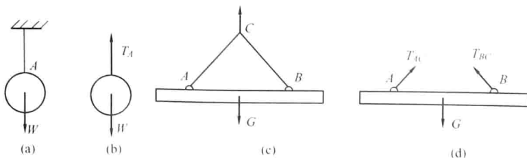
图 1-6 柔索约束及其反力
