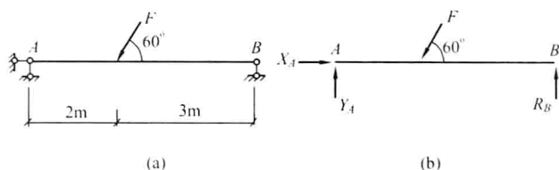
图 1-15 [例 1-1] 图
