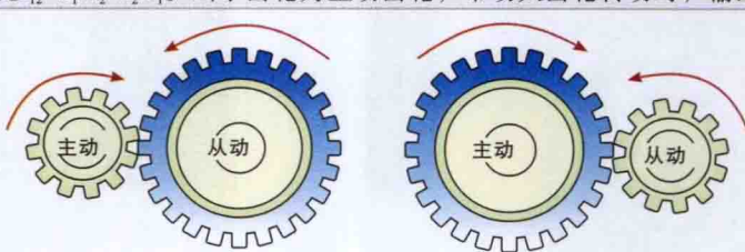
a) 减速传动
