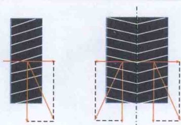
a) 斜齿轮
