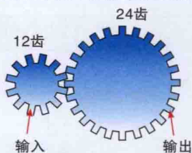
图1 齿轮传动比示意图
