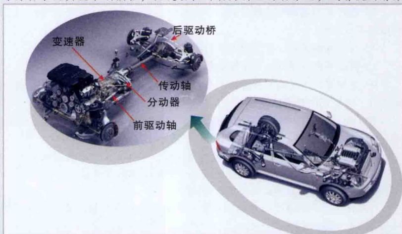
图1 传动系统的组成
