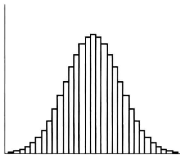
图 1-1 正态分布图
