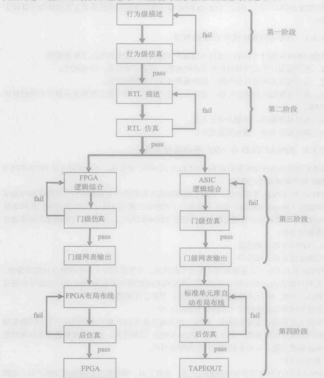
图 1-2 TOP-DOWN 设计流程
