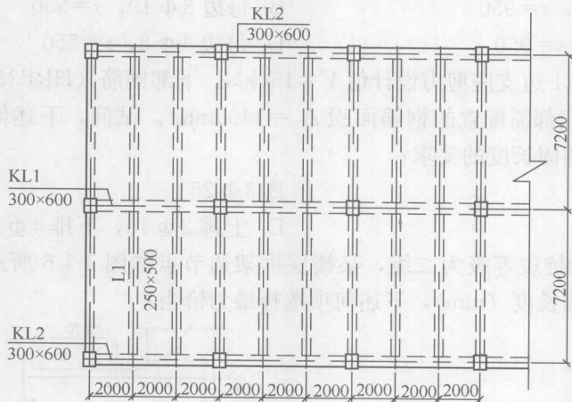
图 1-1-3 题 19~27 图
