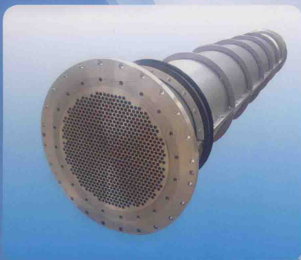
冷却器芯
