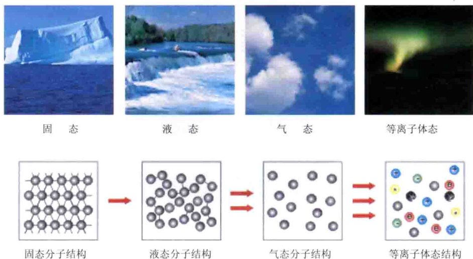
■ 图11-1 物质的四种状态
