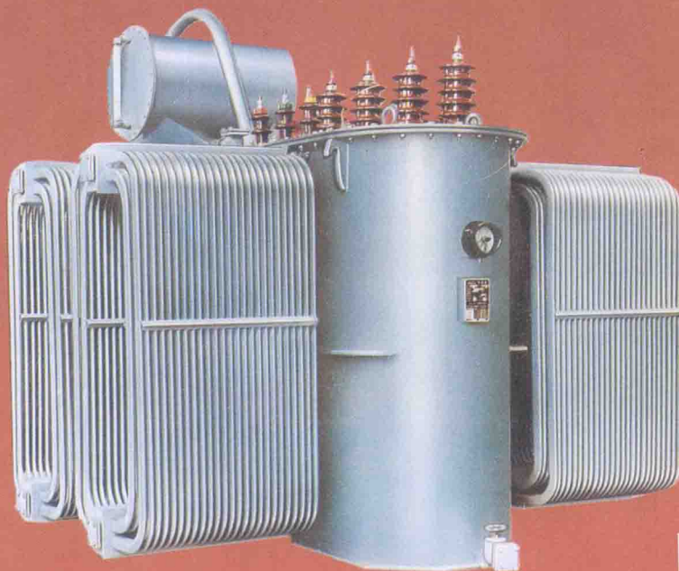
S7—6300KVA/10~0.4 节能变压器
