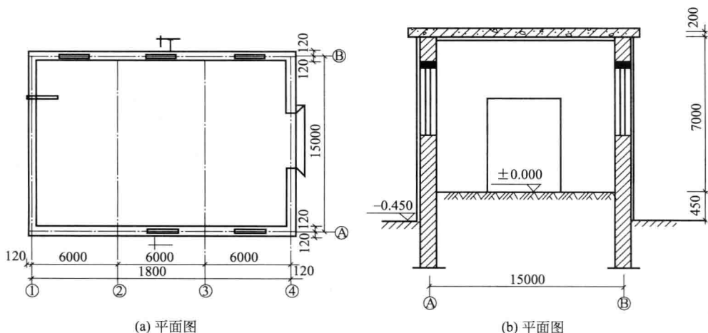
图 1-1 单层仓库
