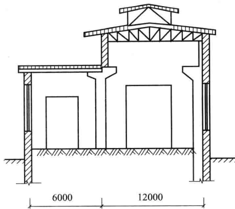
(b) 1—1剖面图
