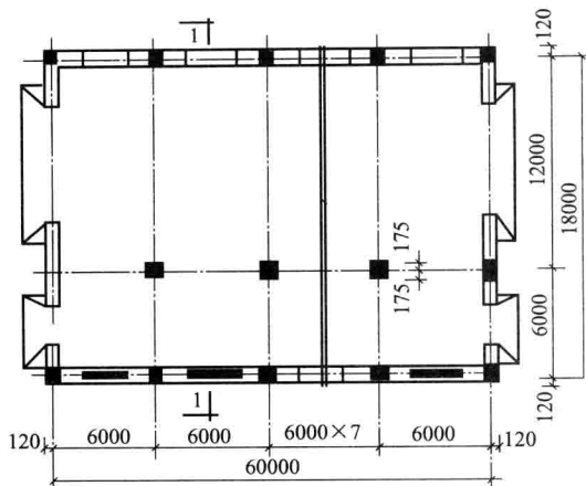
(a) 平面图
