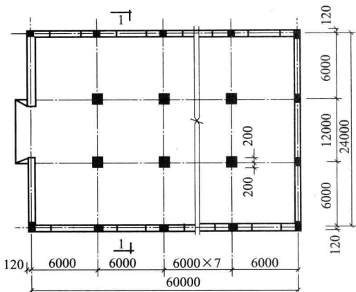
(a) 平面图
