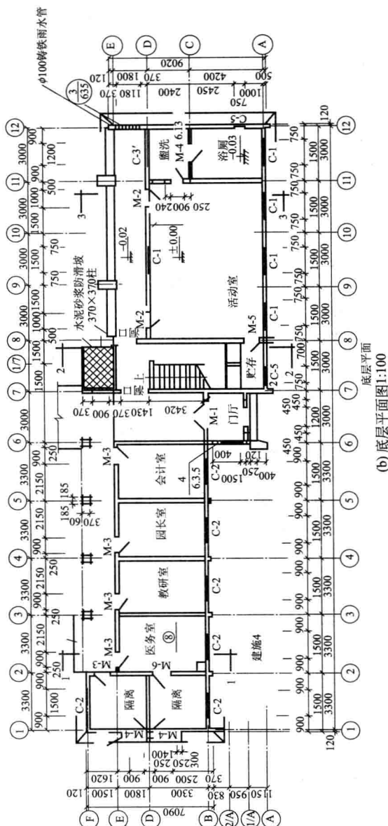
图 1-8 幼儿园底层示意图
