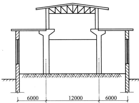
(b) 1—1剖面图
