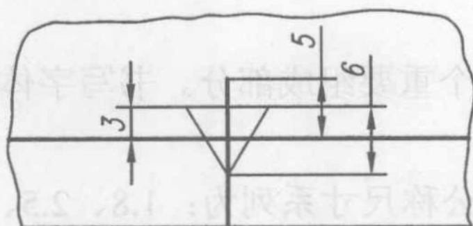
图 1-6 方向符号的大小和位置
