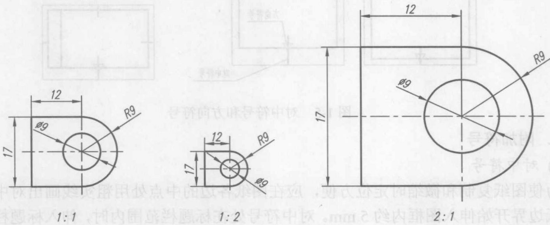
图 1-7 不同比例绘制的图形
