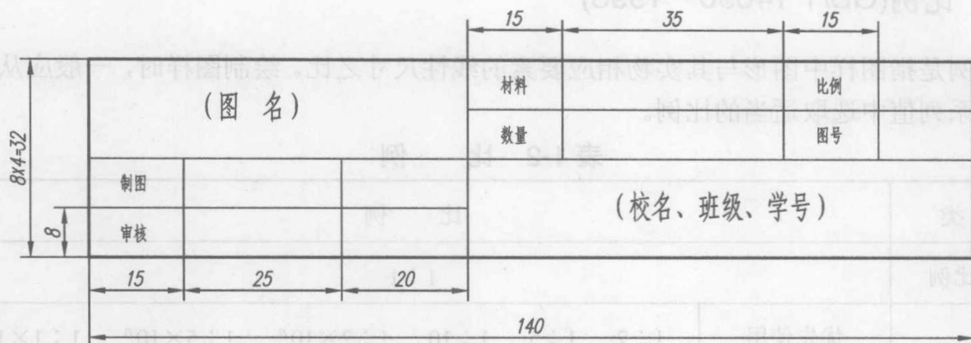
图 1-4 制图作业用标题栏格式
