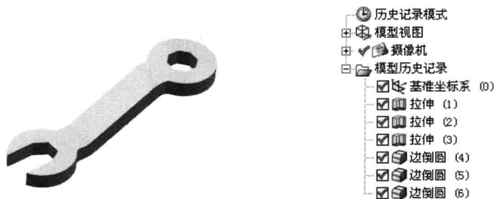
图 1.1 扳手的零件模型及模型树
