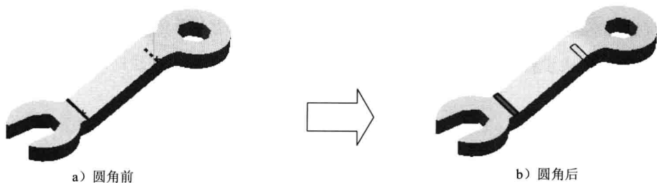
图 1.12 边倒圆特征 3
