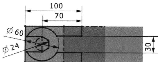
图 1.6 截面草图
