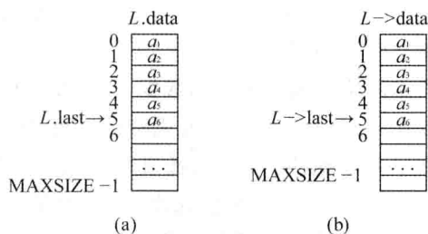
图 1-3 线性表的顺序存储示意图
