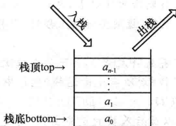
图 1-4 栈的示意图
