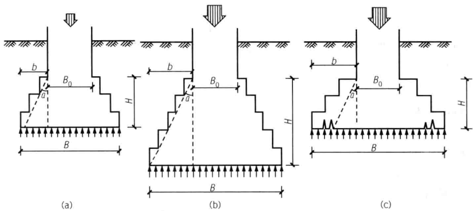
图 1.2-2 刚性基础受力分析
