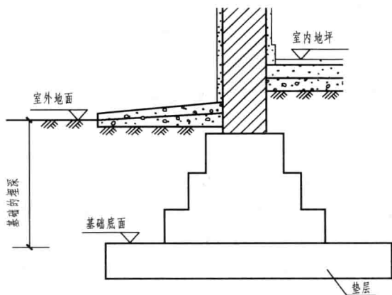
图 1.2-1 基础的埋深
