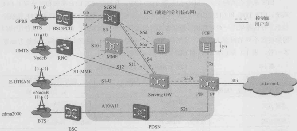
图 1-1 EPS 网络结构
