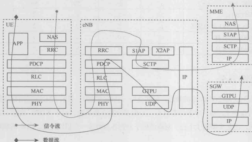
图 1-2 控制面和用户面分离
