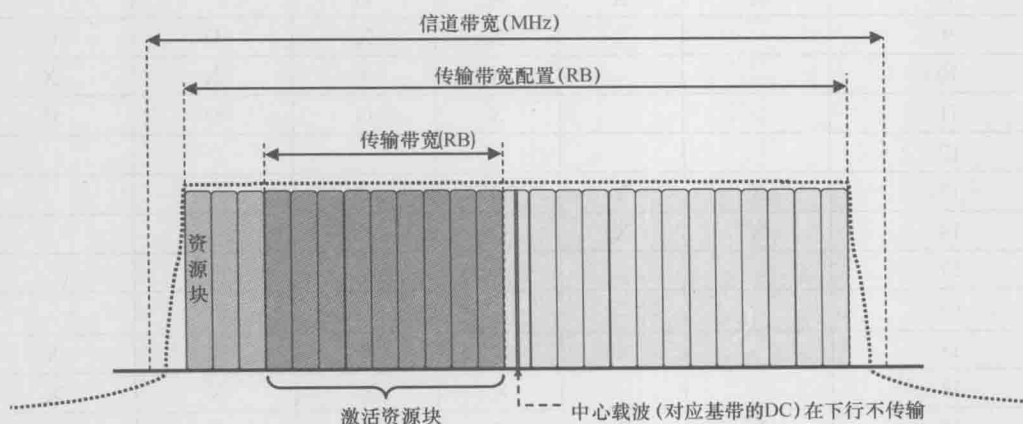
图 1-3 信道带宽和传输带宽配置的定义
