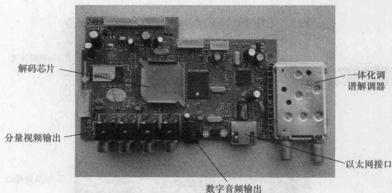
主电路板
