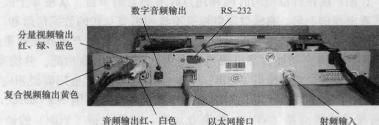
背面接口
