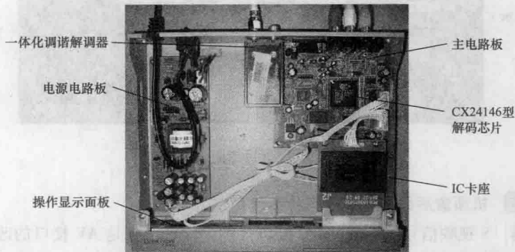
内部电路结构
