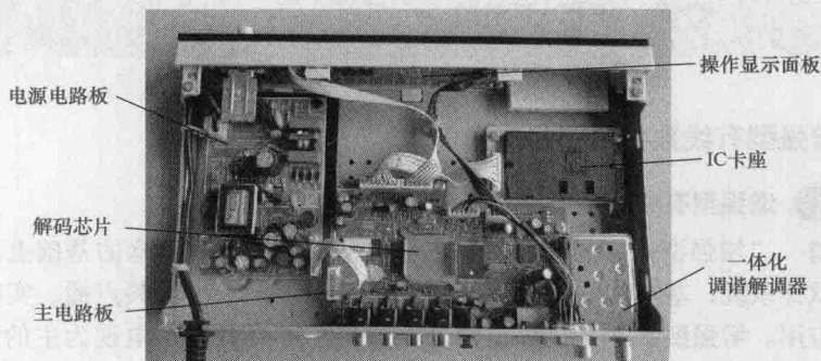
内部结构
