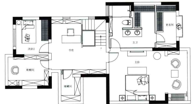
二层平面布置图
