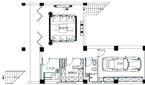
一层平面布置图
