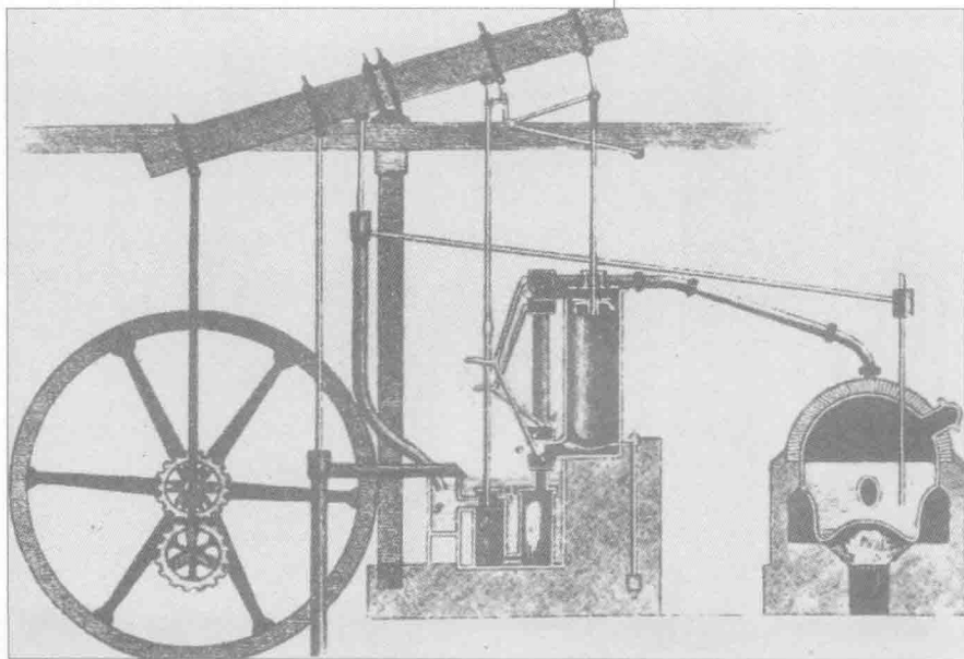
■詹姆斯·瓦特发明的蒸汽机
