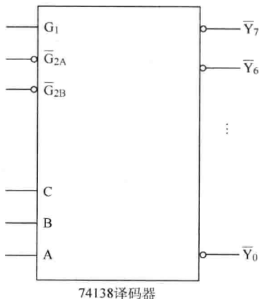
图 1-2 常用的 3-8 译码器
