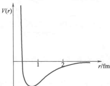
图 0-2 核力示意图
