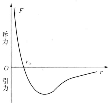
图 9-2 分子间的相互作用力
