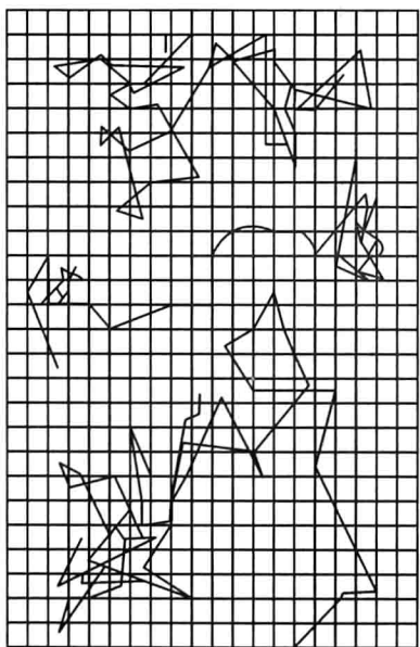
图 9-1 布朗运动
