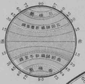
緯線及回歸線
