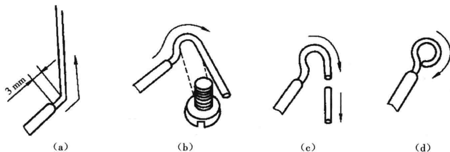
图 1-19 单股芯线羊角圈弯法
