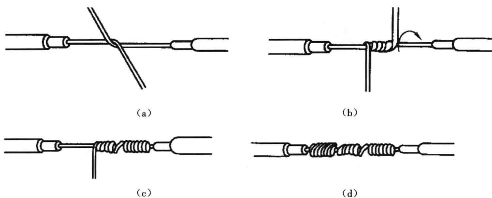
图 1-13 单股铜芯导线直接连接
