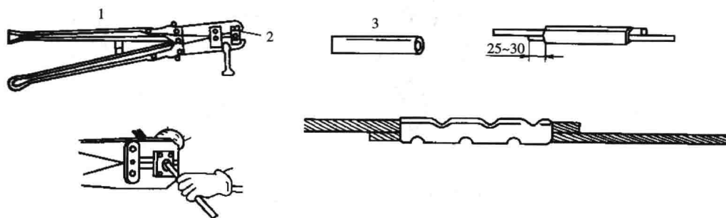
图 1-17 钳接管压接法
