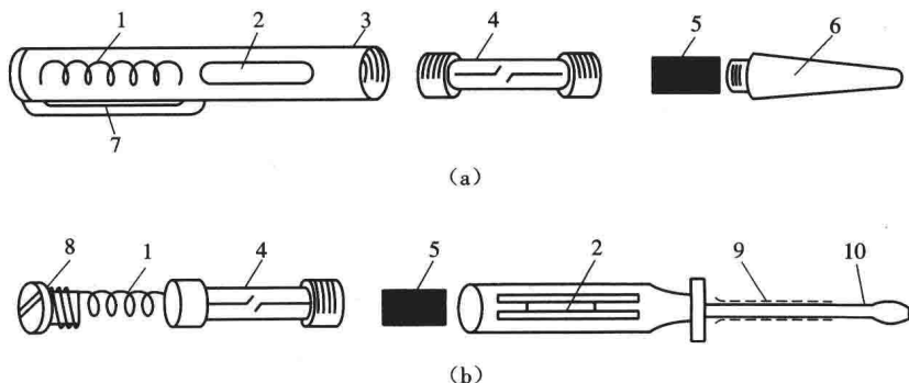
图 1-1 验电笔结构
