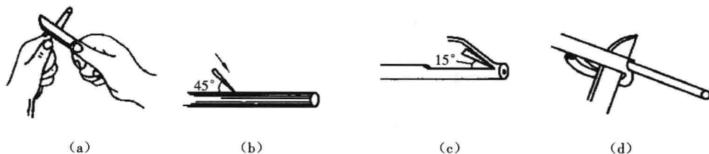
图 1-10 电工刀剥离塑料硬线绝缘层
