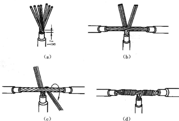
图 1-16 股铜芯导线的 T 形分支连接
