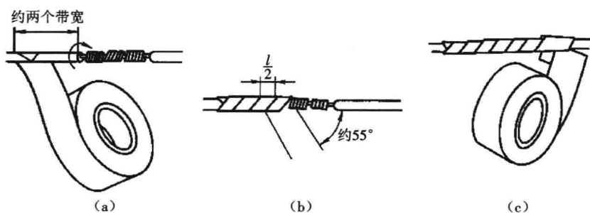
图 1-21 绝缘带的包缠方法
