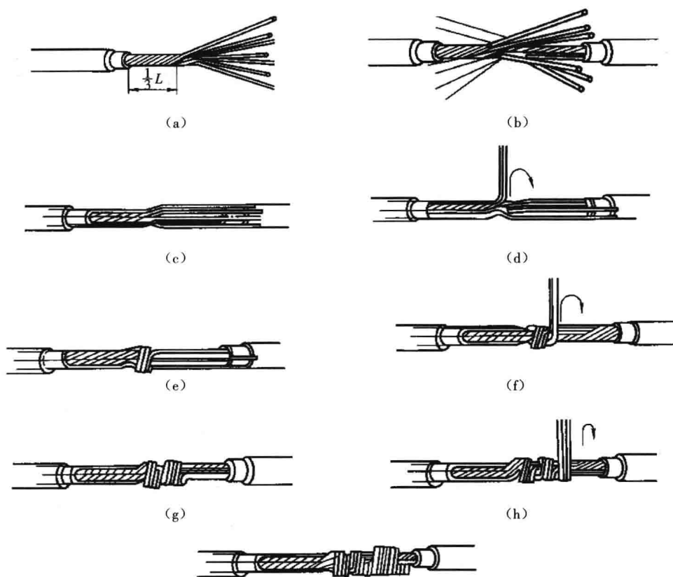
图 1-15 股铜芯导线的直接连接
