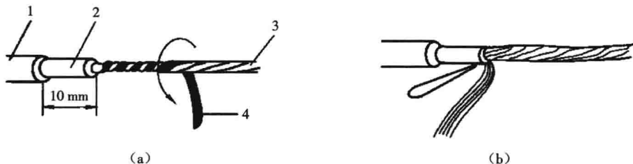
图 1-12 花线绝缘层的剖削
