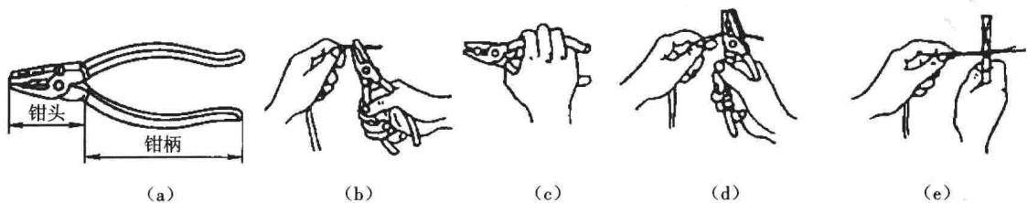
图 1-2 钢丝钳构造及其使用方法
