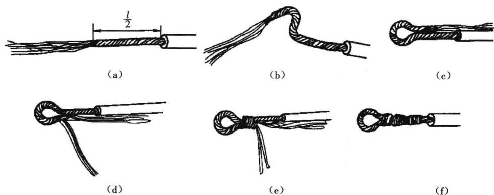
图 1-20 多股芯线压接圈弯法
