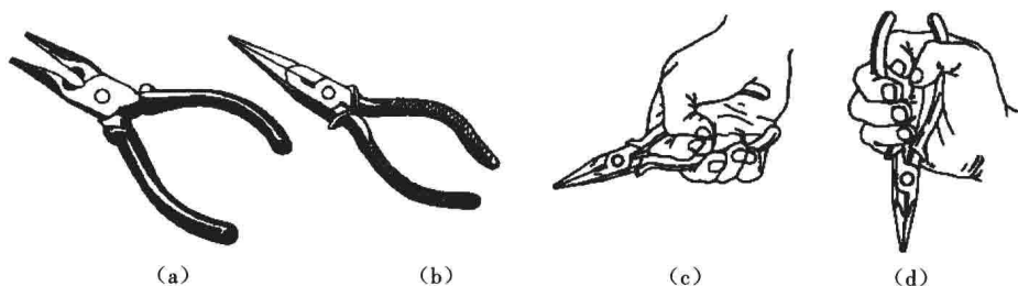
图 1-3 尖嘴钳外形结构及使用方法
