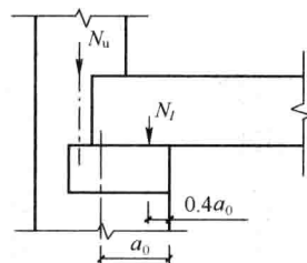
图 4.2.5 梁端支承压力位置
