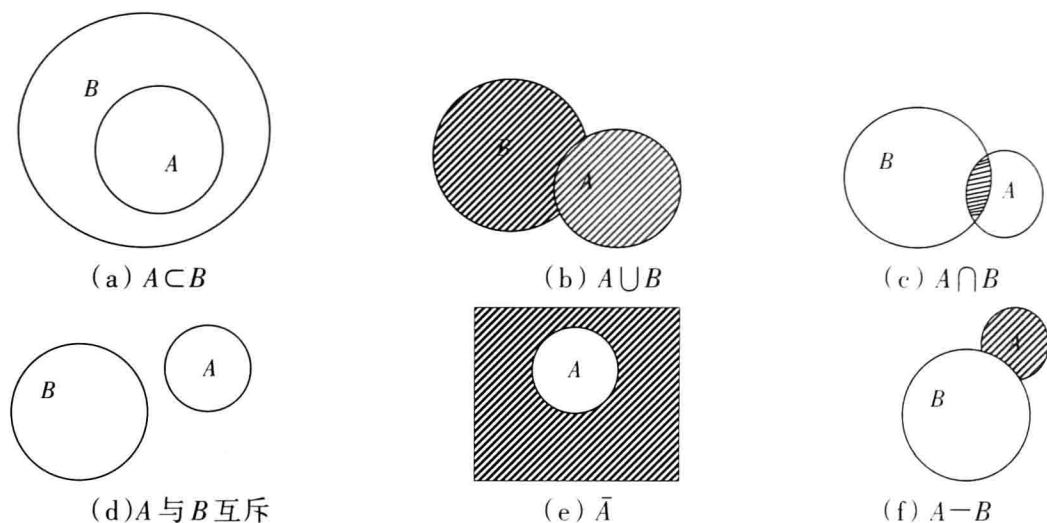
图 1-1 维恩(Venn)图
