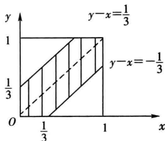
图 1-2 会面问题
