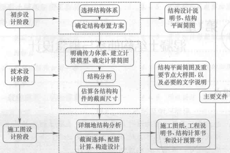
图 1-1 混凝土结构设计一般程序流程图
