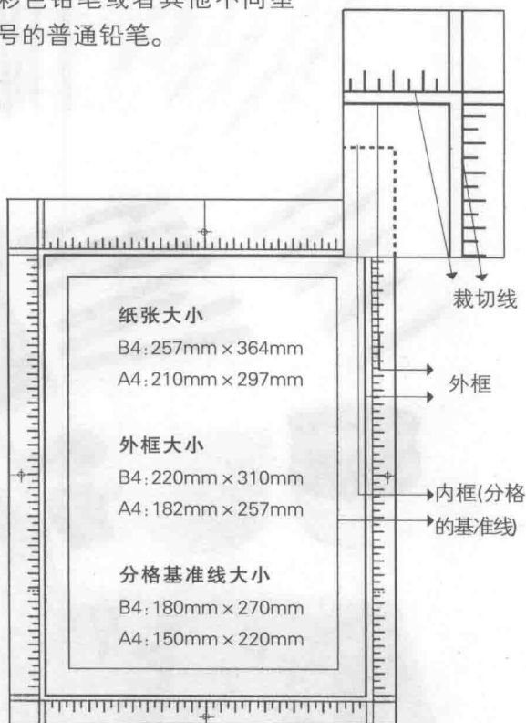
漫画原稿纸
