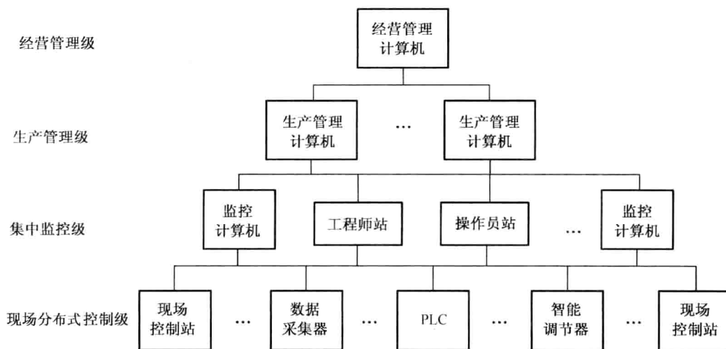
图 1.8 计算机分级分布式控制系统
