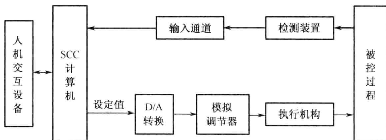
图 1.6 SCC + 模拟调节器控制系统
