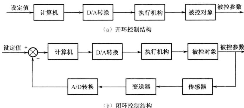
图 1.2 计算机控制系统
