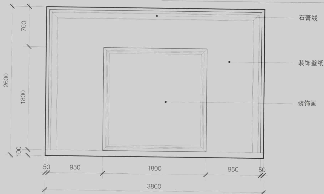
倒边镜斜拼
