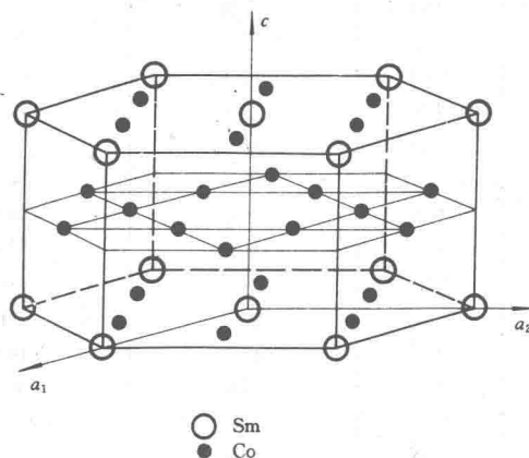
图 21-4 \text{CaCu}_5 型晶体结构图 ( \text{RECo}_5 )
