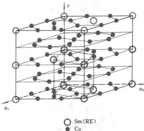
图 21-5 \text{Th}_2\text{Ni}_{17} 型晶体结构图 ( \text{RE}_2\text{Co}_{17} )
