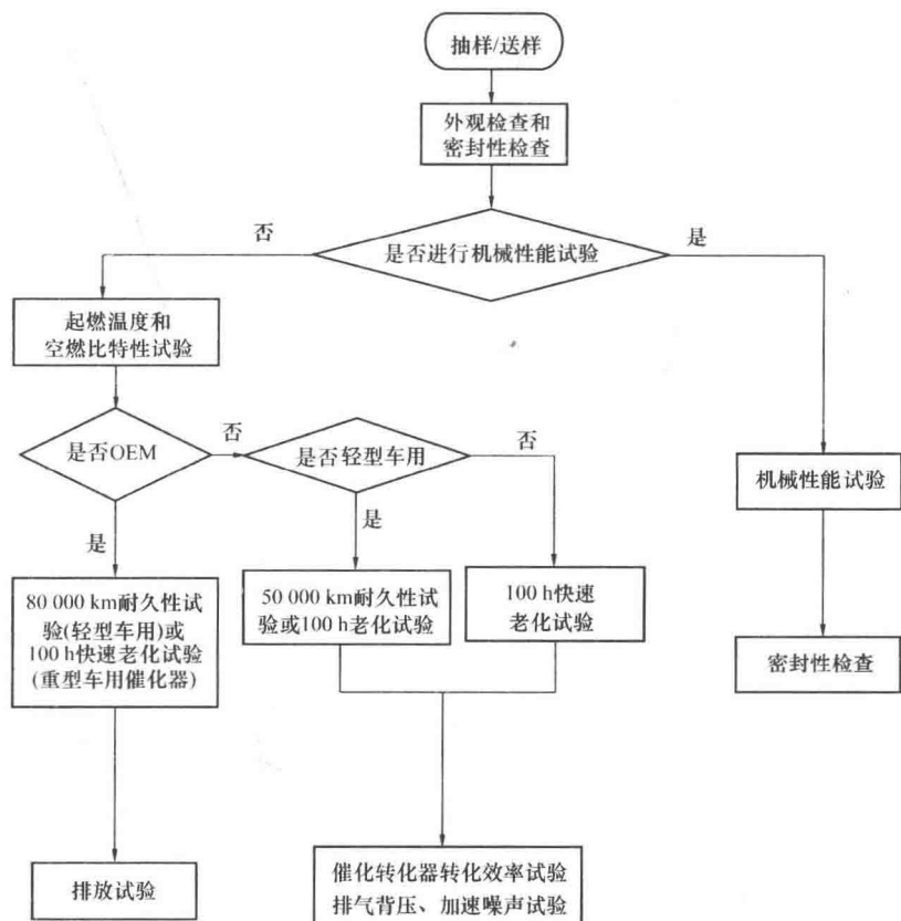
图 1 催化转化器试验程序图
