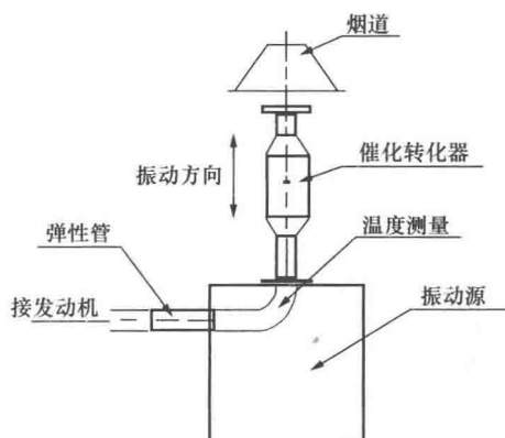
图3 纵置热振动试验安装示意图
