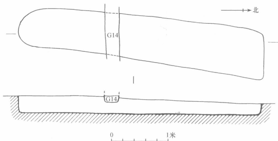
图七 H42平、剖面图
