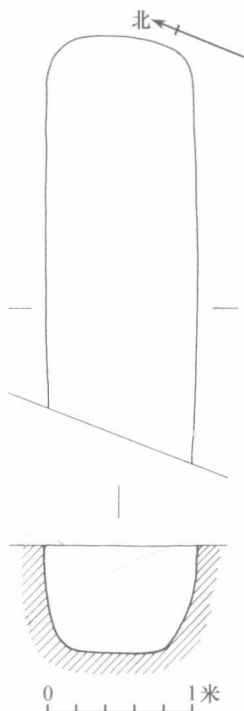
图八 H65平、剖面图
