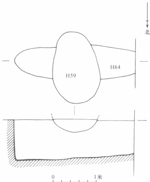
图九 H59、H64平、剖面图
