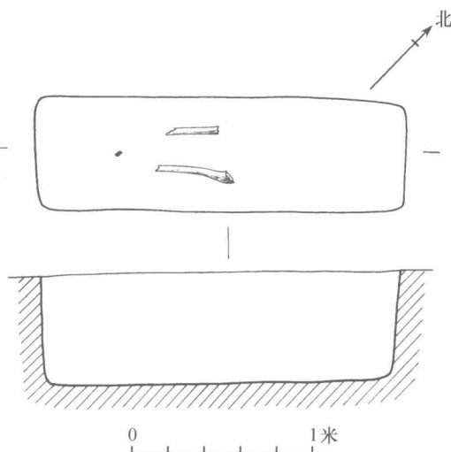
图一六 M2平、剖面图
