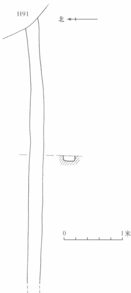
图一二 G14平、剖面图
