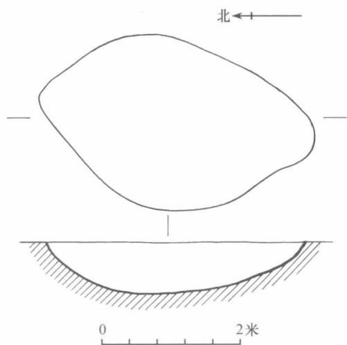
图一一 H58平、剖面图
