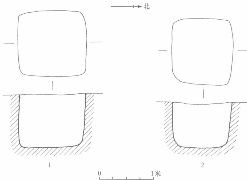
图一四 F1柱坑平、剖面图
