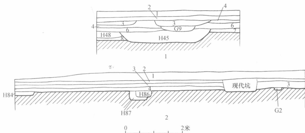
图三 探方剖面图
