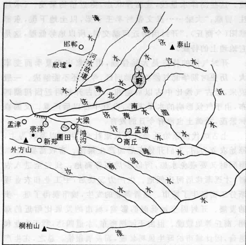
上古开封附近水系图(战国时代)
