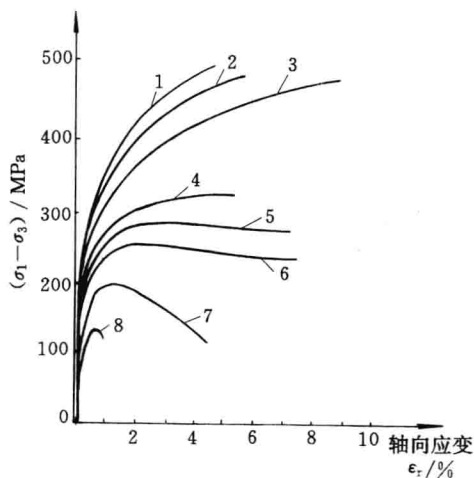
图 1-2 大理岩单轴和三轴应力—应变全过程图
