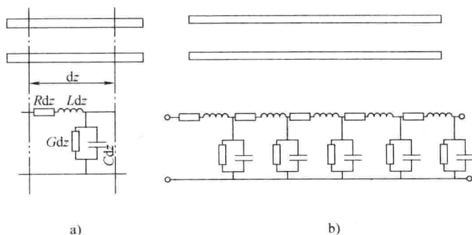
图 1-1 传输线的电路模型
