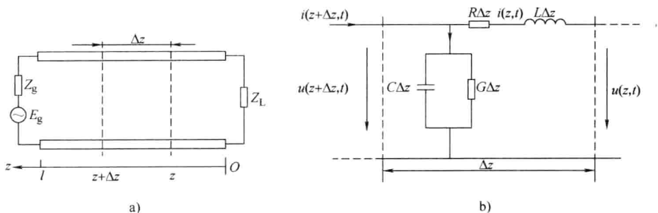
图 1-2 均匀传输线及其等效电路
